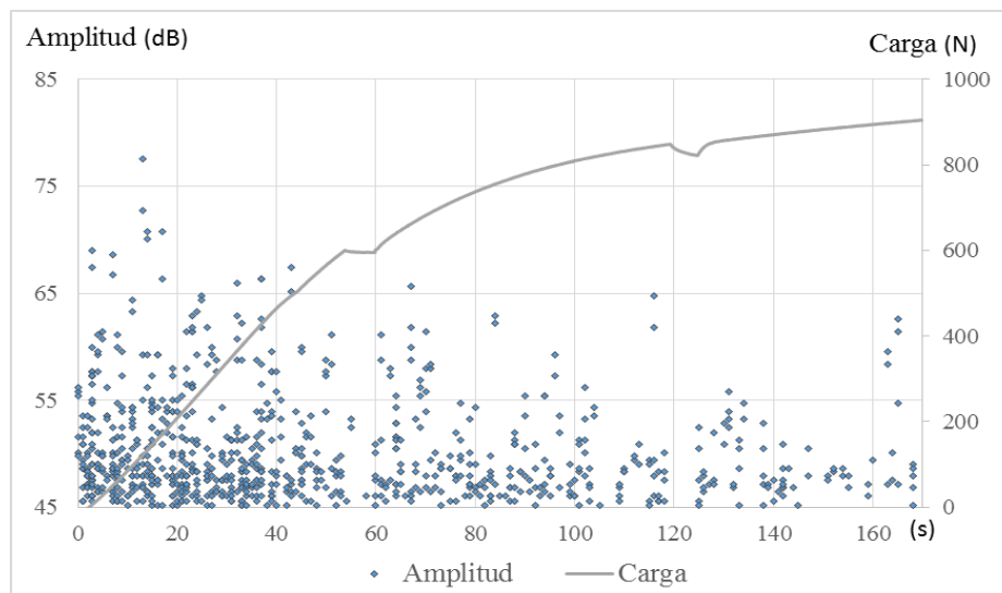
Figura 6. Superposición de amplitud de eventos y fuerza Vs tiempo probeta R1B.
