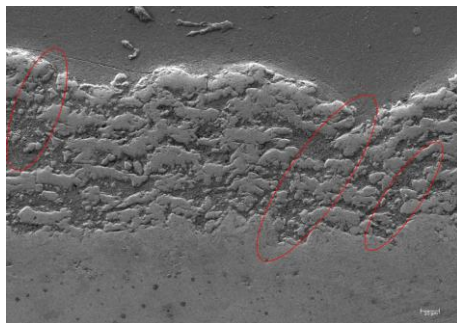
Figura 13. a) SEM grietas superficiales Serie S X250 b) SEM corte transversal serie S x500.
