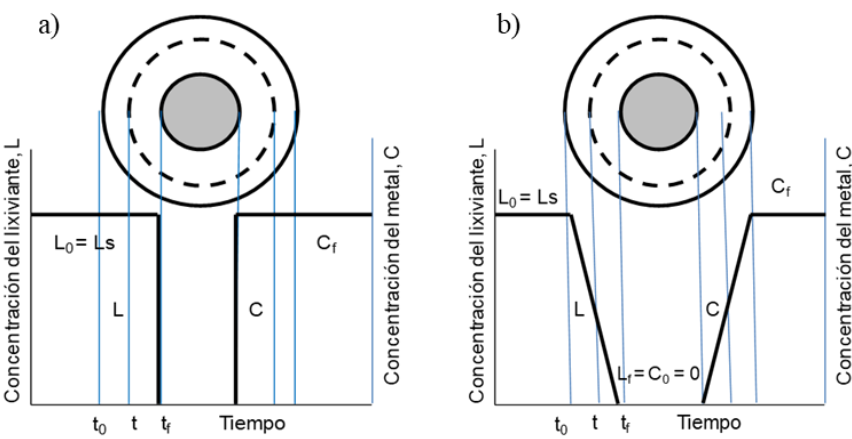
Figura 5. Modelo de núcleo sin reaccionar con control por a) reacción química y b) difusión en la capa de producto.
