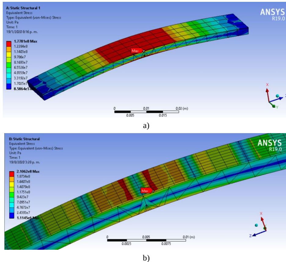
Figura 15. Simulación por elementos finitos a) placa con recubrimiento continuo b) placa con recubrimiento segmentado.
